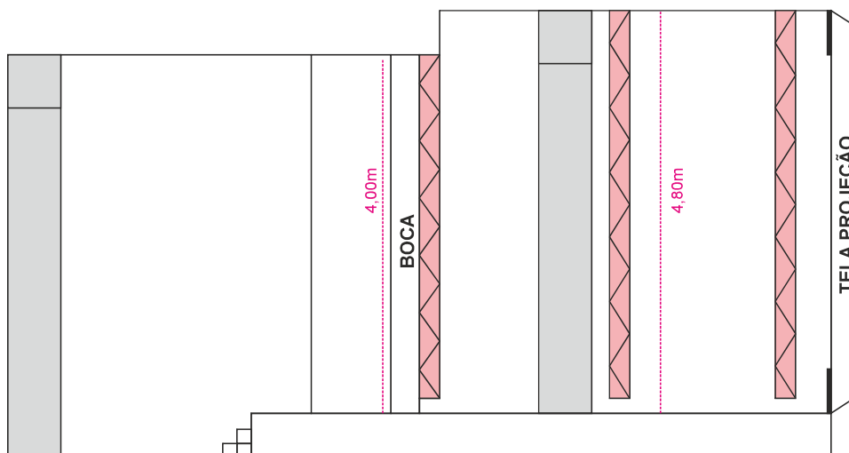
VISTA LATERAL PALCO (DIMENSÕES)
